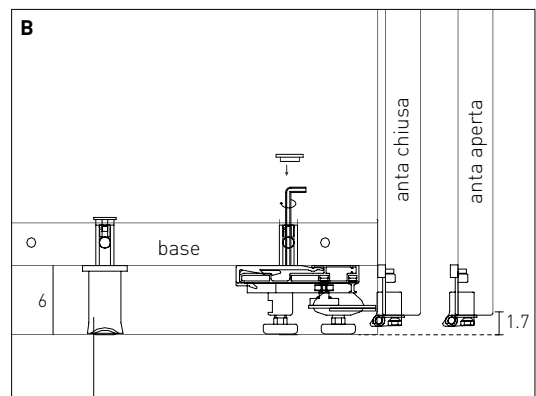
piedino livellatore (regolazione max 1 cm)
