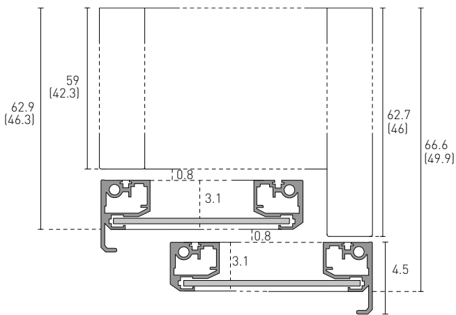
Profondità armadio complanare con fianco Sp 3 senza cornice
