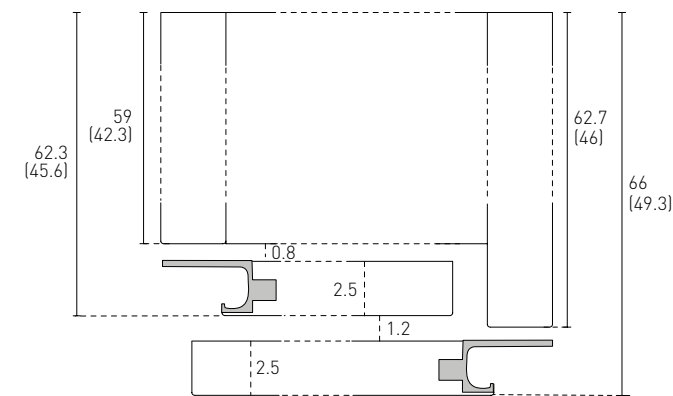
Profondità armadio complanare (per ante con vetro aumentare la P di cm 0.3) con fianco Sp 3 senza cornice
