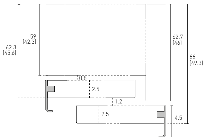
Profondità armadio complanare con fianco Sp 3 senza cornice
