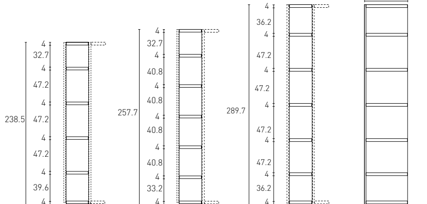
Terminale con ripiani vista frontale
