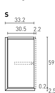
Terminale a scrigno (no H 289.7)
