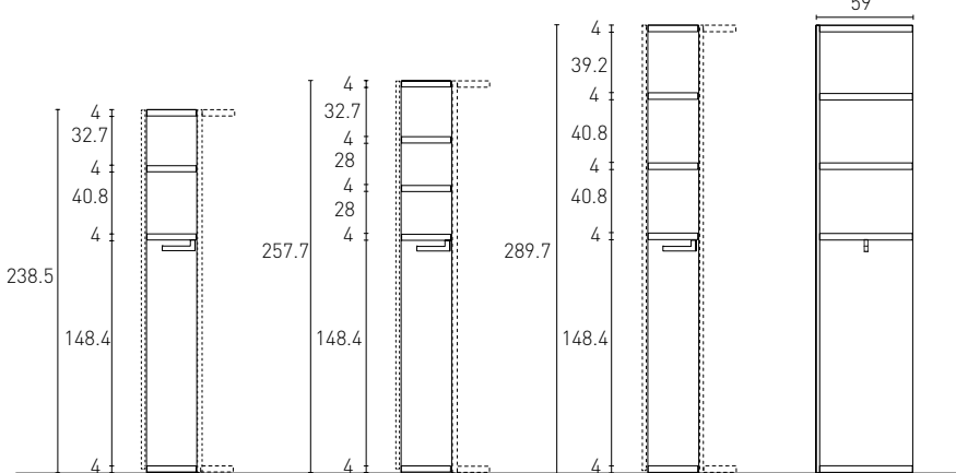
Terminale con ripiani tipo A vista frontale
