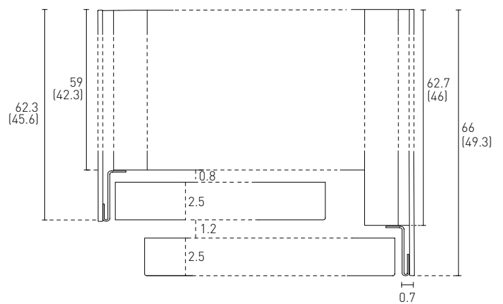
con fianco di finitura Sp 3.9
