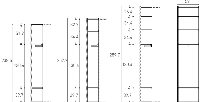
Terminale con ripiani tipo B vista frontale
