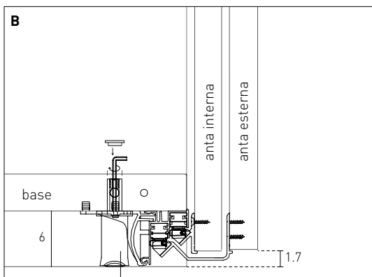
piedino livellatore (regolazione max 1 cm)
