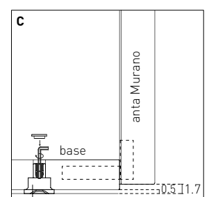
piedino livellatore (regolazione max 1 cm)
