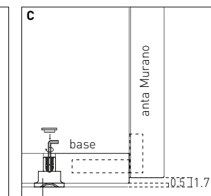
piedino livellatore (regolazione max 1 cm)
