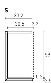
Terminale a scrigno (no H 289.7)
