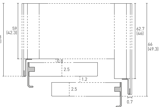
con fianco di finitura Sp 3.9
