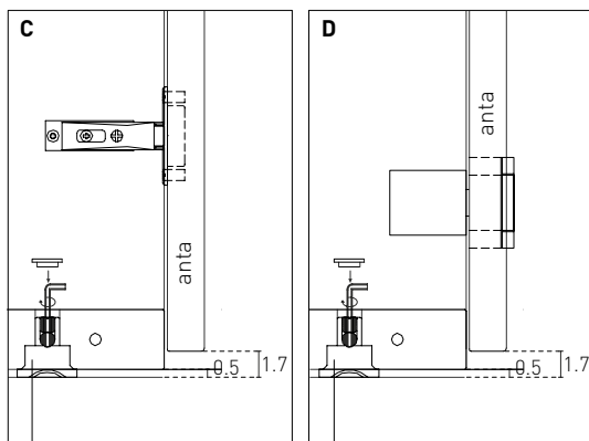
pedino livellatore (regolazione max 1 cm)
