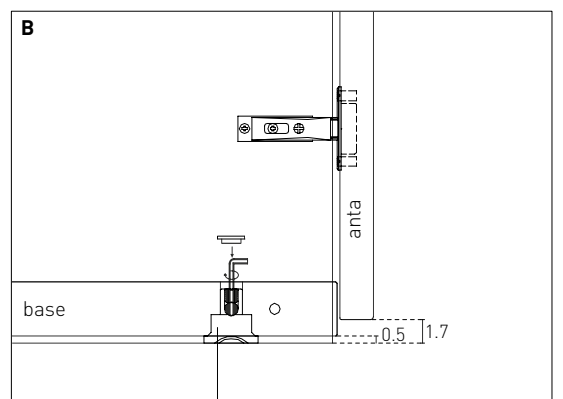
pedino livellatore (regolazione max 1 cm)
